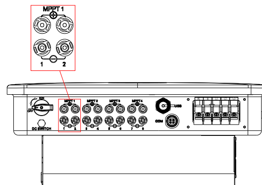
图 5.5 PV端子
