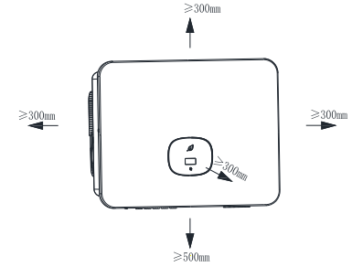
图4.2 一台逆变器时安装尺寸
