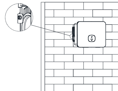
图 4.8 逆变器壁挂示意图
