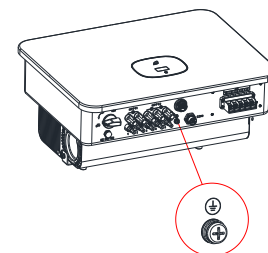
图 5.1 接地示意图
