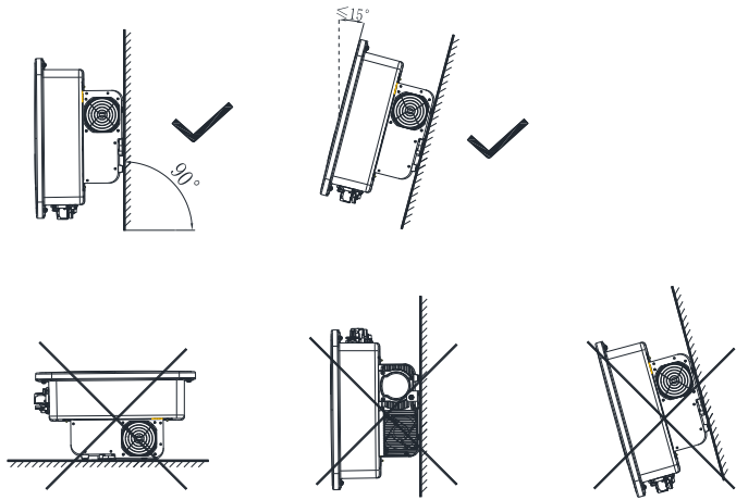
图 4.1 安装示意图
