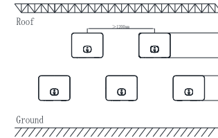
图 4.3 多台逆变器时的安装尺寸
