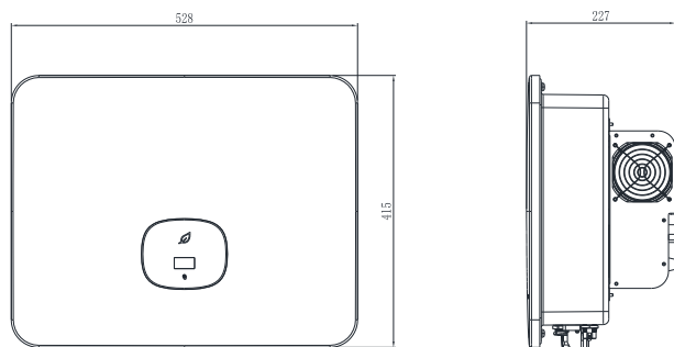
图 2.2 尺寸规格
