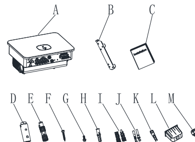
图 3.1 配件图
