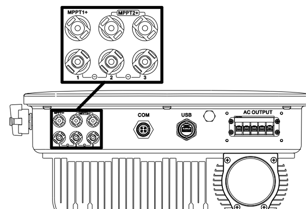
图 5.5 PV端子
