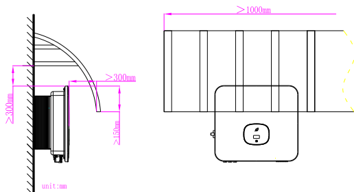
图 4.6 遮阳棚
