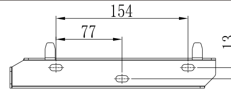
图 4.7 壁挂架规格图
