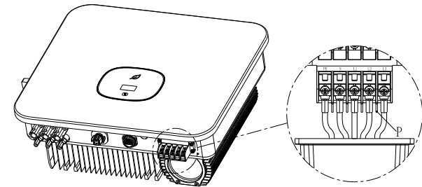
图 5.3 AC端子接线示意
