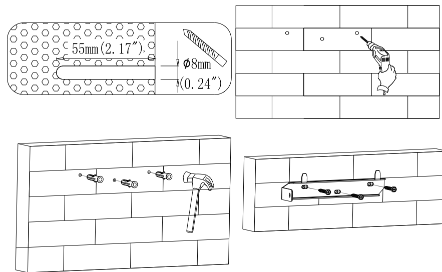
图 4.8 壁挂架安装示意图
