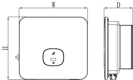
图 2.2 尺寸规格
