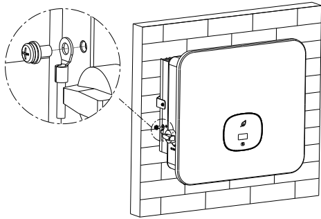
图 5.1 接地示意图
