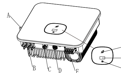
图 2.1 外观概图
