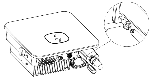
图 5.4 AC端锁防水罩示意
