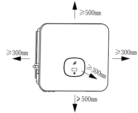
图 4.2 一台逆变器时安装尺寸
