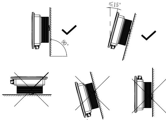
图 4.1 安装示意图
